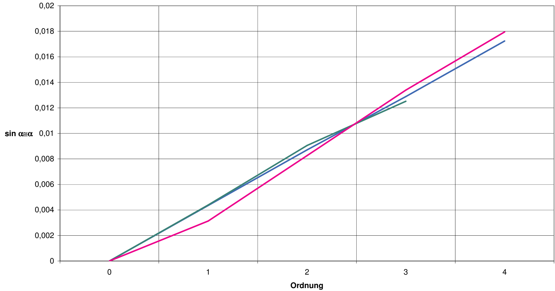
Diagramm 1 Ablenkung der Minima in Abhängigkeit von der Ordnung
