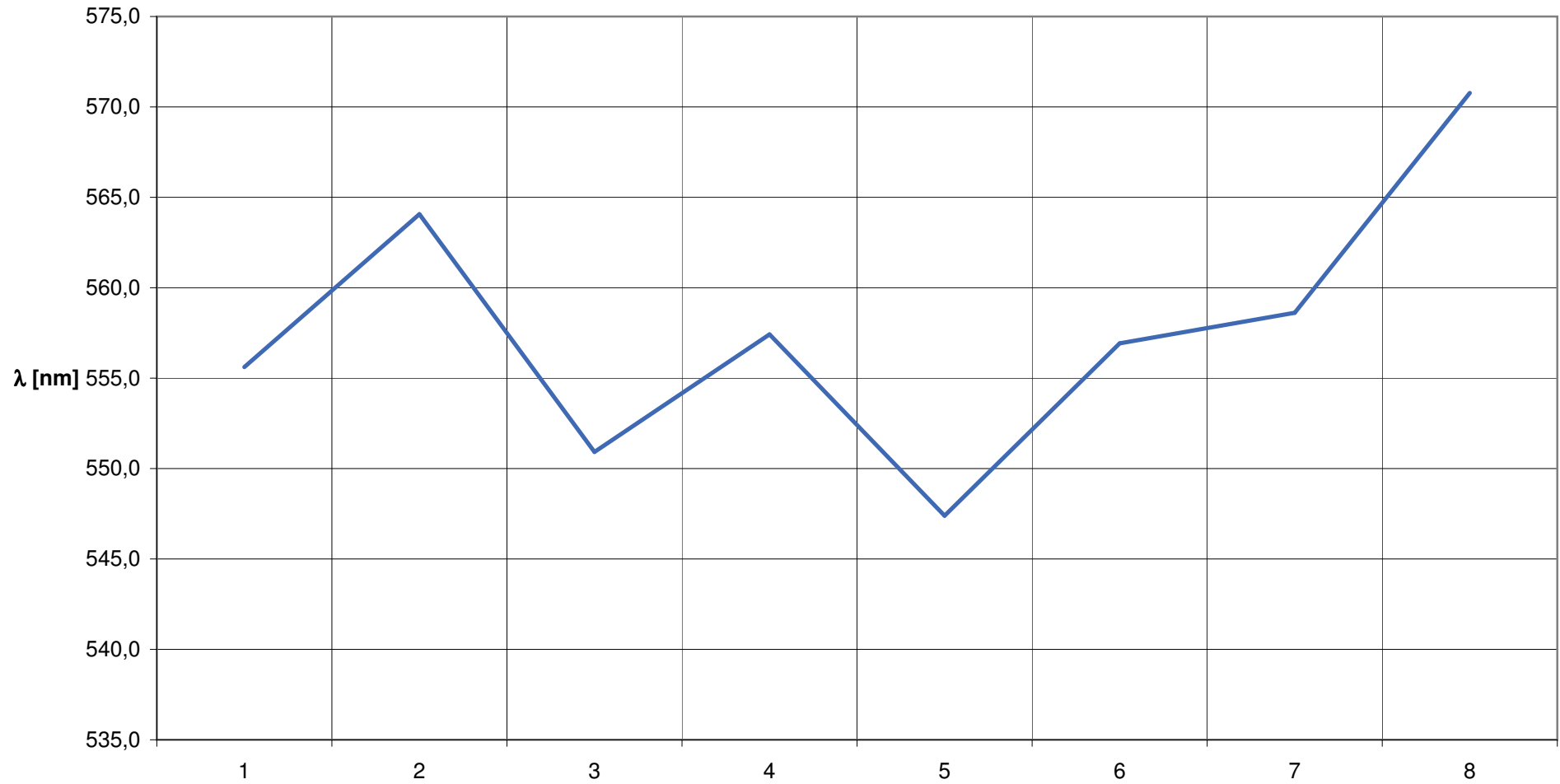
Diagramm 4 Wellenlänge (Mittelwerte) der grünen Spektrallinie des Quecksilbers in Abhängigkeit der Maxima/Minima
