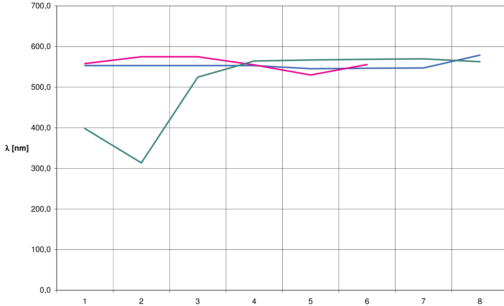
Diagramm 3 Wellenlänge der grünen Spektrallinie des Quecksilbers in Abhängigkeit der Maxima/Minima
