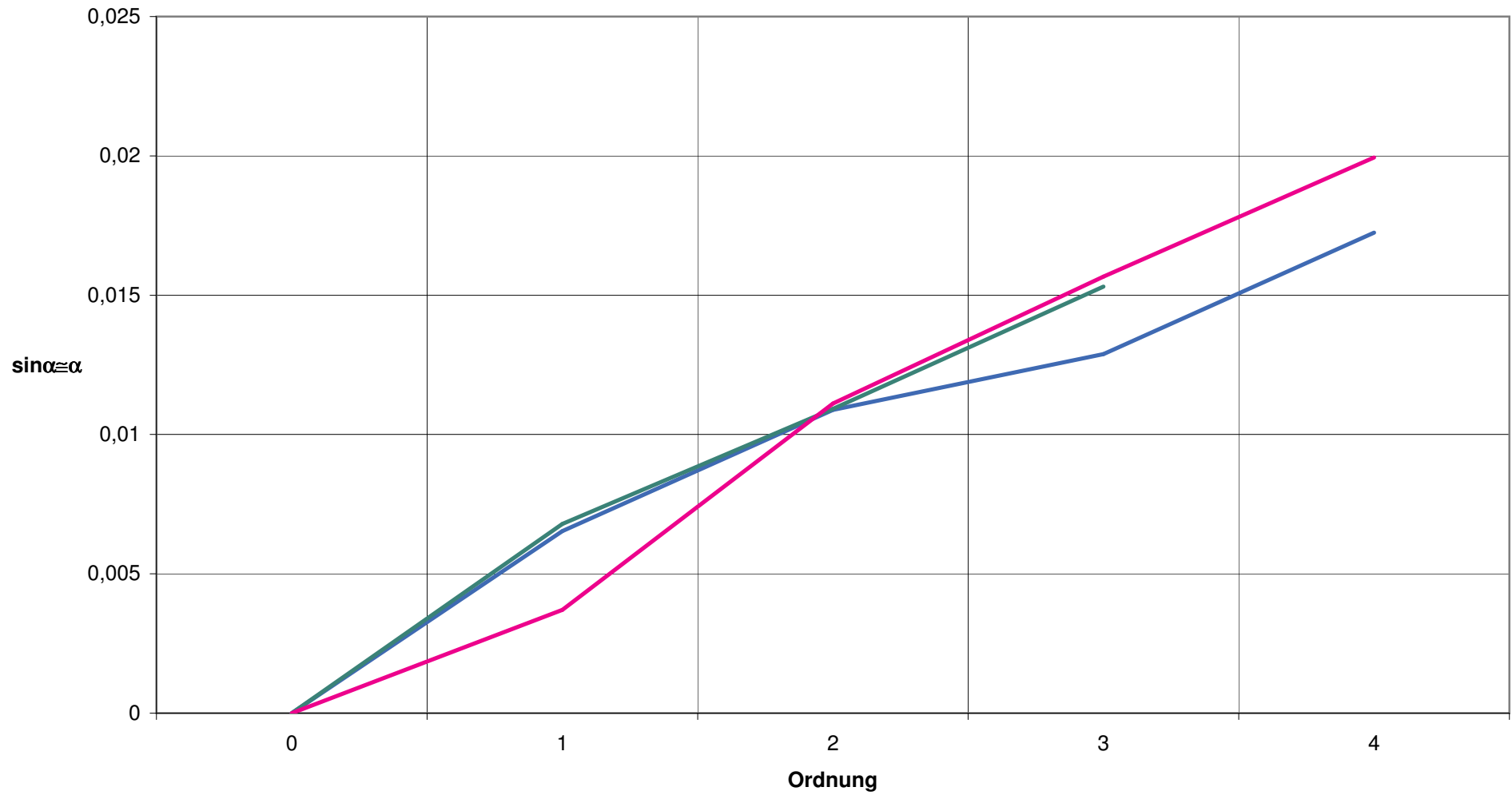
Diagramm 2 Ablenkung der Maxima in Abhängigkeit von der Ordnung
