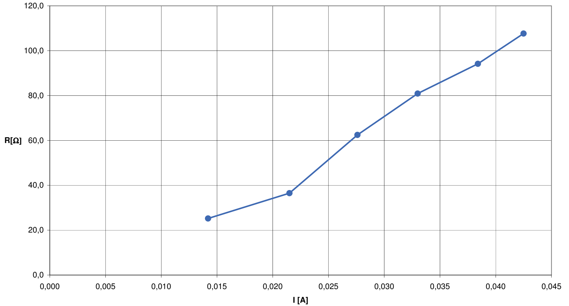
R_{\text{Glühbirne}} [\Omega] (vergl. R = 10 )
