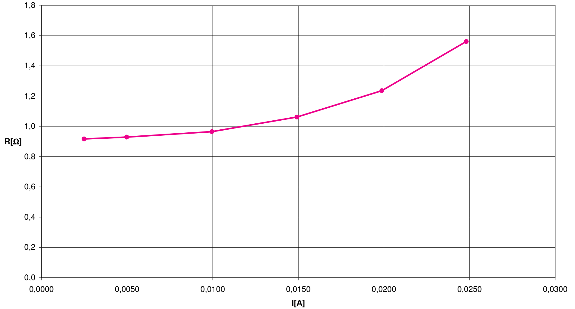
R_{\text{Glühbirne}} [\Omega] (vergl. R = 200 )
